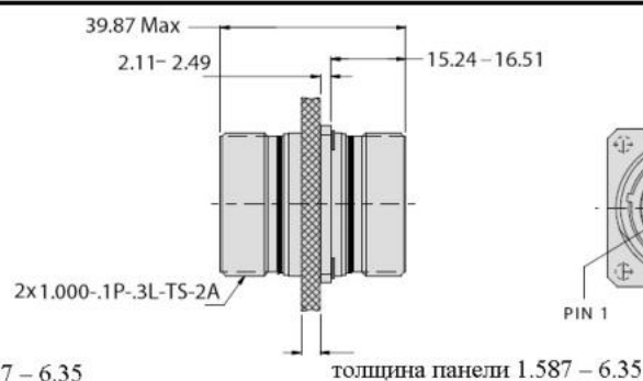
переходники, тип CM
