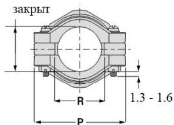
увеличенный кабельный зажим закрыт
