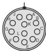
контактная схема 19 - 11
