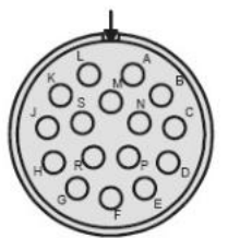
контактная схема 21 - 16
