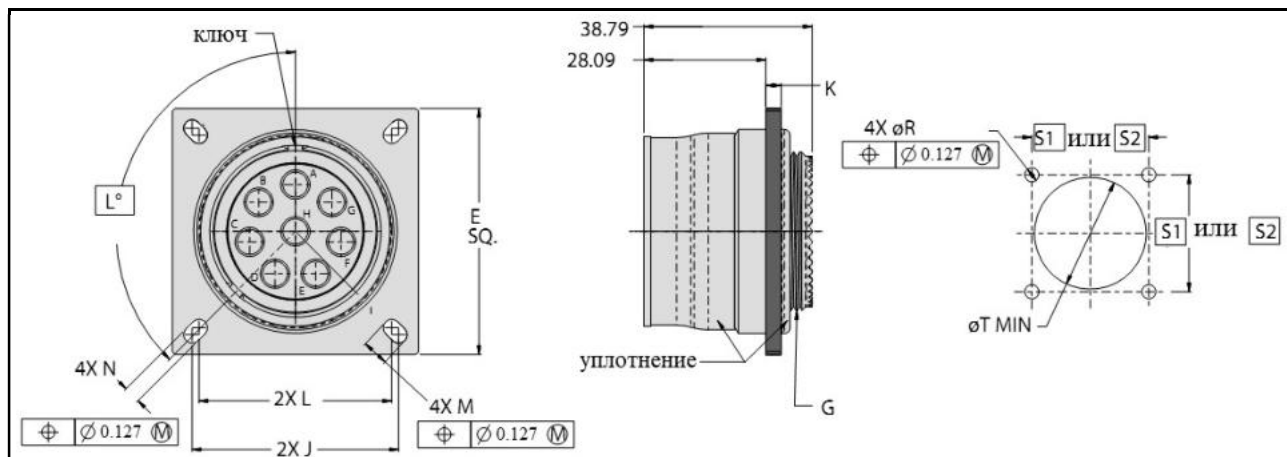
Розетки, тип 253-045-00, с уплотнениями
