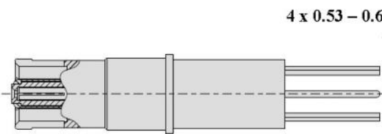
гнездовой контакт
