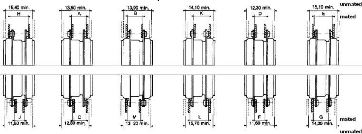
Толщина установочной панели
