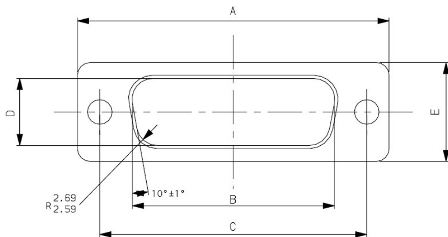
Вид сочленяемой стороны
