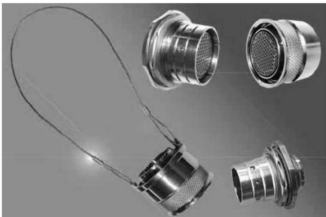
Серия 8D Соединители с системами сочленения Push – Pull и Quick release MIL-DTL-38999, серия 3
