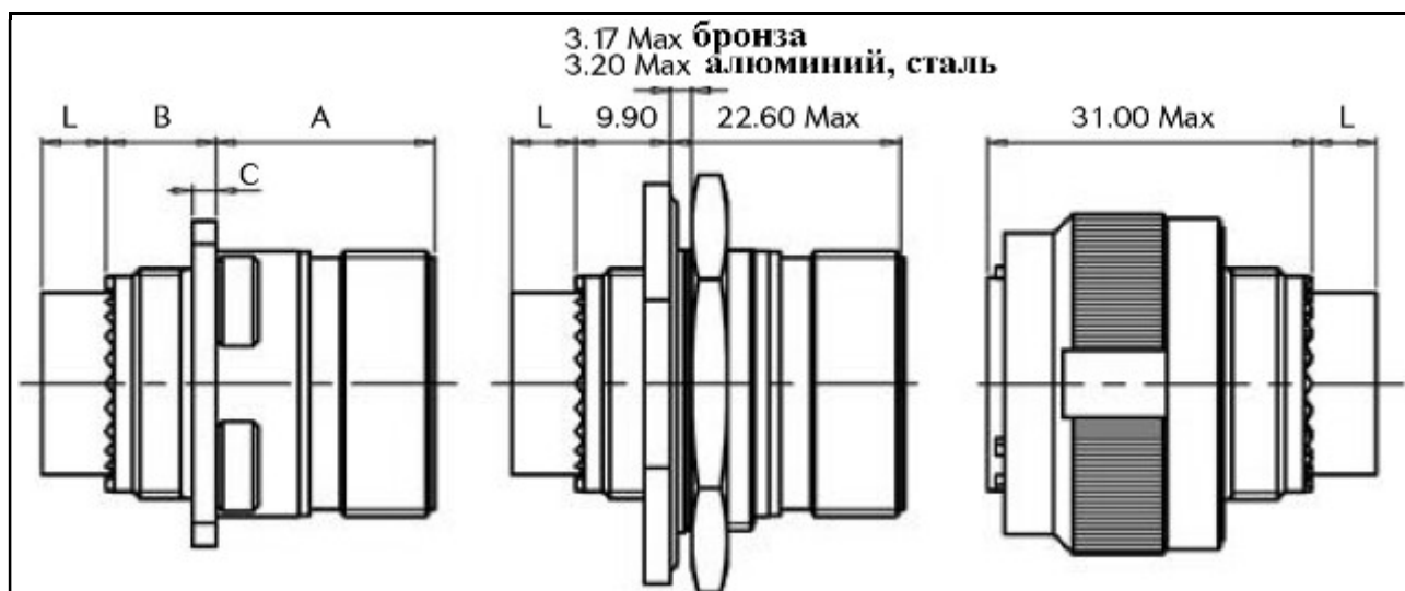
Розетка, тип 0
