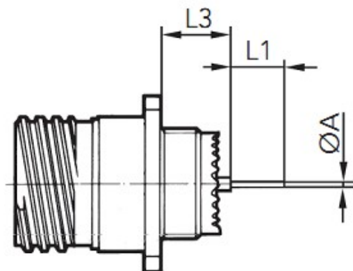
розетка, тип 00
