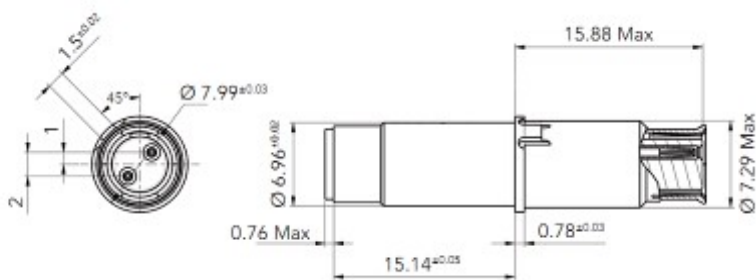
гнездовой контакт
