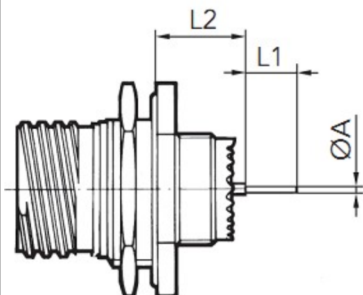
розетка, тип 07
