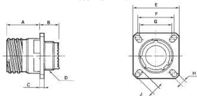
Розетка тип 0
