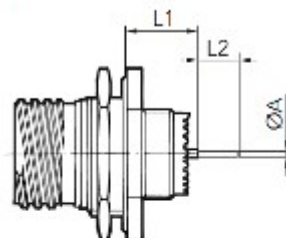
розетки, тип 7
