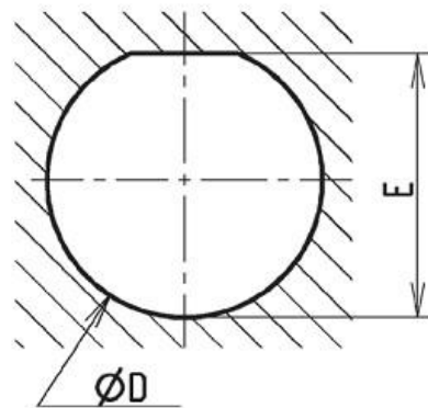
под крепление контргайкой
