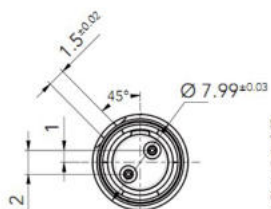
Твинаксиальные контакты под обжимку
