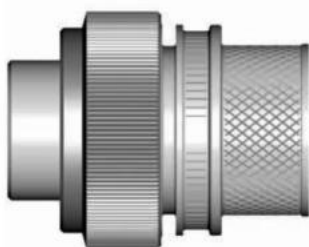
D1: прямой кожух под установку ТУТ или экрана (обжимные контакты)
