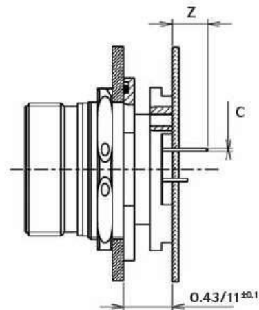
Розетка с дв. фланцем 8D8711
