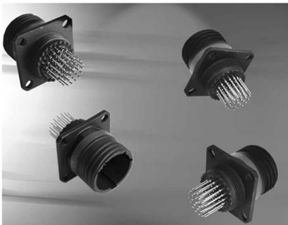
Серия 8D Соединители герметизированного типа MIL-DTL-38999, серия 3
