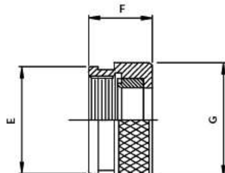
Кожух под ТУТ (несъёмный наконечник) тип 60-2G
