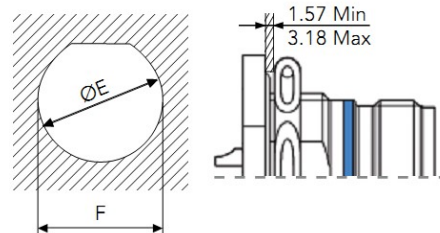
Розетки, тип 7Y/7YE
