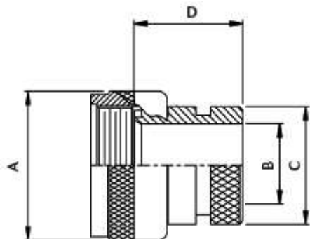
Кожух под ТУТ (съёмный наконечник) тип 60-1
