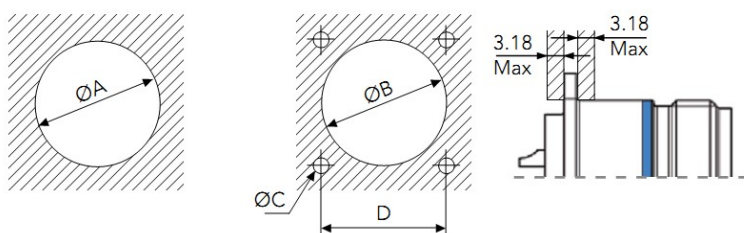
Розетки, тип 2Y/2YE
