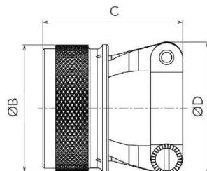
Прямой кожух
