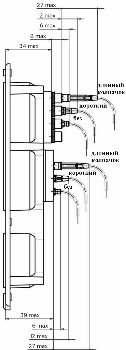
Розетка ARINC600
