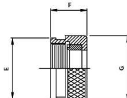
Кожух под ТУТ (несъёмный наконечник) тип 60-2G
