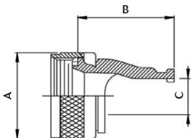
Прямой кожух тип 53
