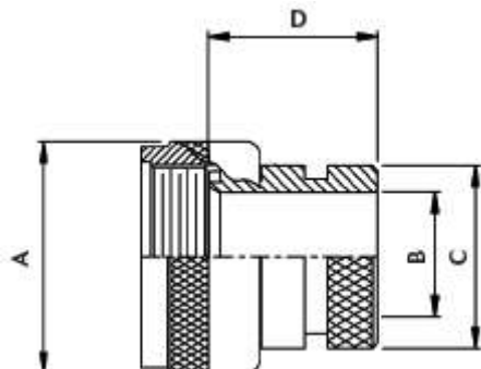
Кожух под ТУТ (съёмный наконечник) тип 60-1
